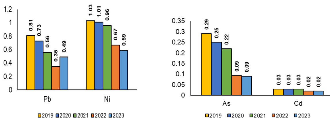
4.2. attēls. Gada vidējā svina, niķeļa, arsēna un kadmija koncentrācija nokrišņos, µg/l novērojumu stacija “Rucava”
