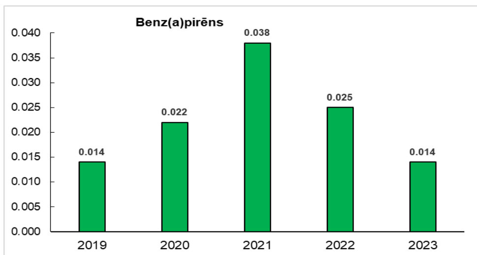
4.6. attēls. Benz(a)pirēna kopējais nosēdumu daudzums lauku fona stacijā “Rucava” 2019.-2023.g., \mu\text{g}/\text{m}^3 \times \text{dienā}
