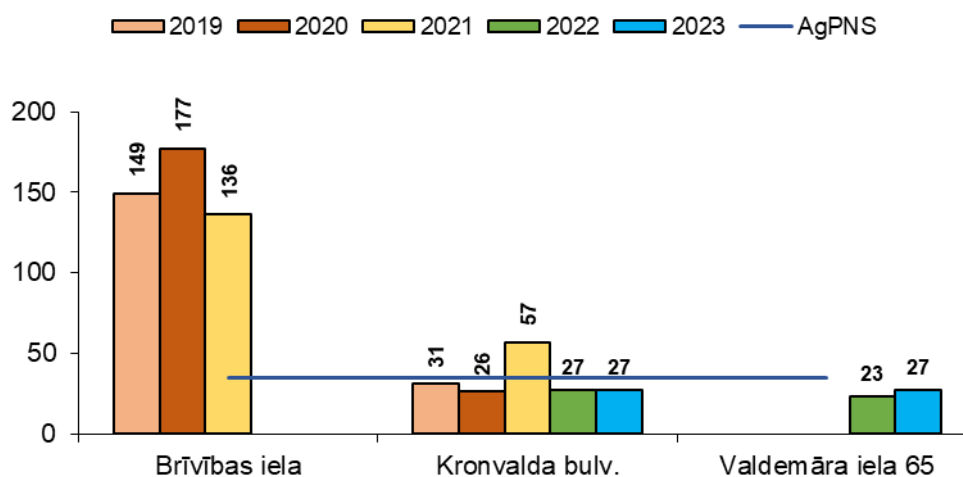
2.8. attēls. Daļiņu PM 10 diennakts AgPNS pārsniegšanas gadījumu skaits, Rīgā.
