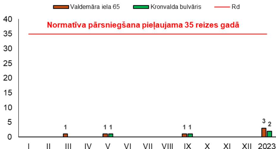
2.7. attēls. Daļiņu PM 10 diennakts koncentrācijas pārsniegšanas gadījumu skaita dinamika mēnešu griezumā stacijās Rīgā, 2023.g.
